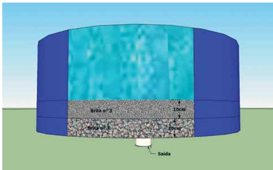
Corte do Filtro
