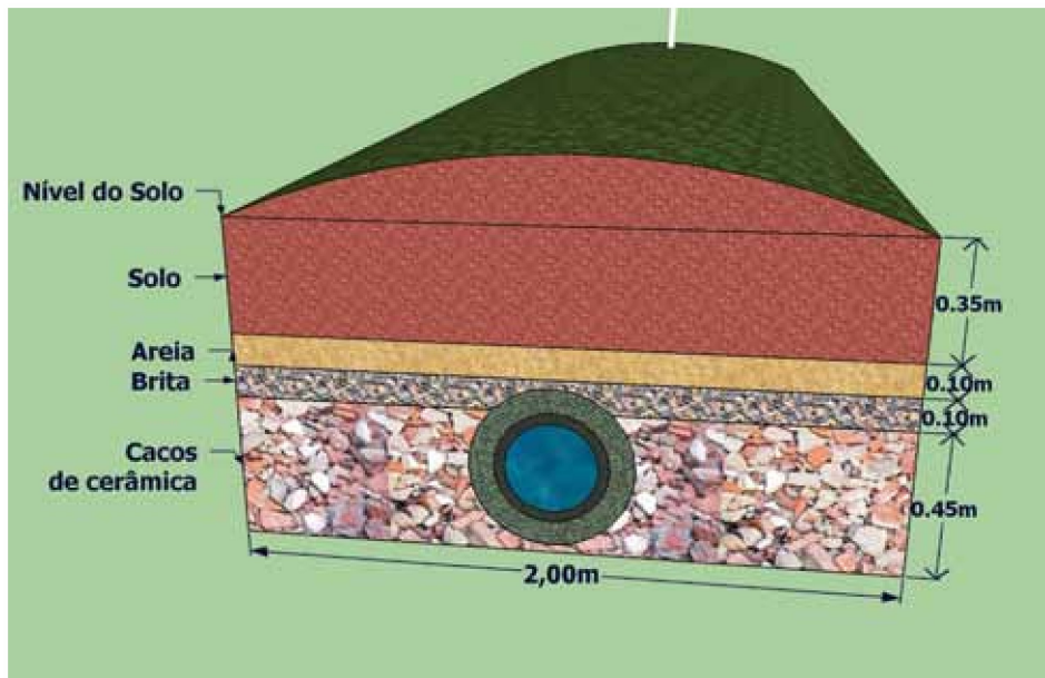
Corte esquemático de um Tevap
