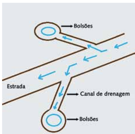
Sistema de drenagem de estradas
