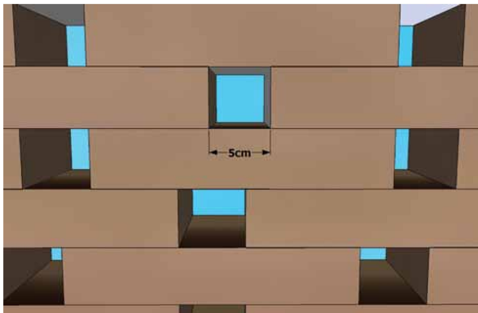
Detalhe da parede de infiltração
