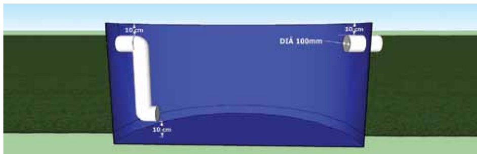
Dimensões da fossa biodigestora
