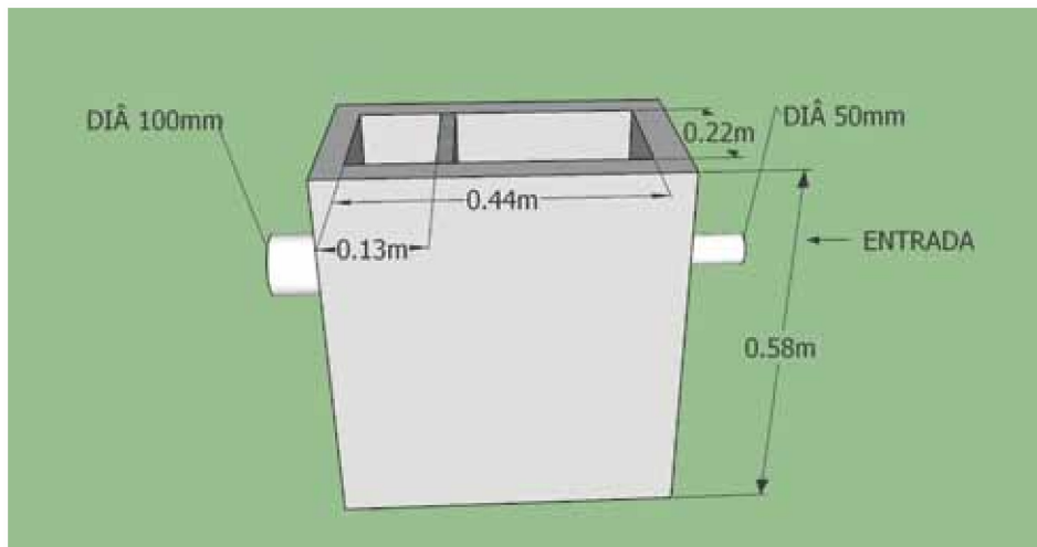
Dimensões mínimas de caixa de gordura
