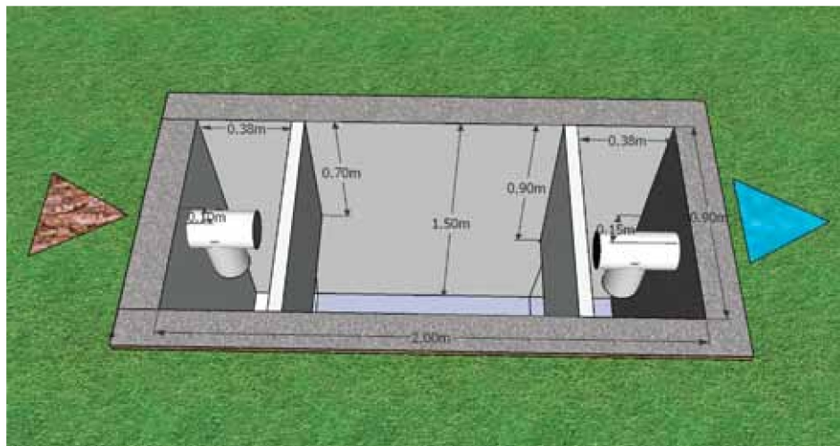
Dimensionamento de uma fossa séptica retangular para família com até 7 pessoas
