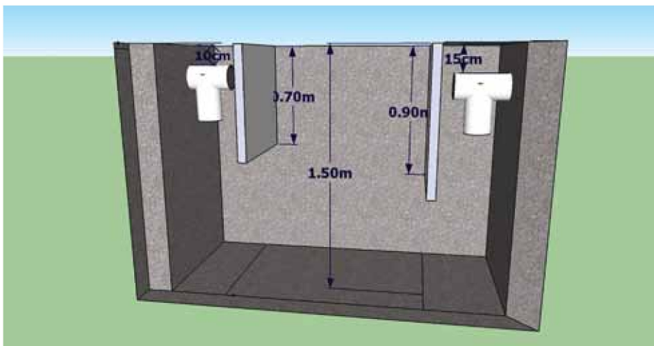
Vista lateral de fossa séptica retangular para 7 pessoas
