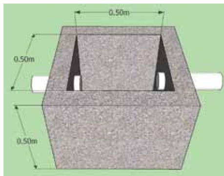
Caixa de inspeção para fossa séptica
