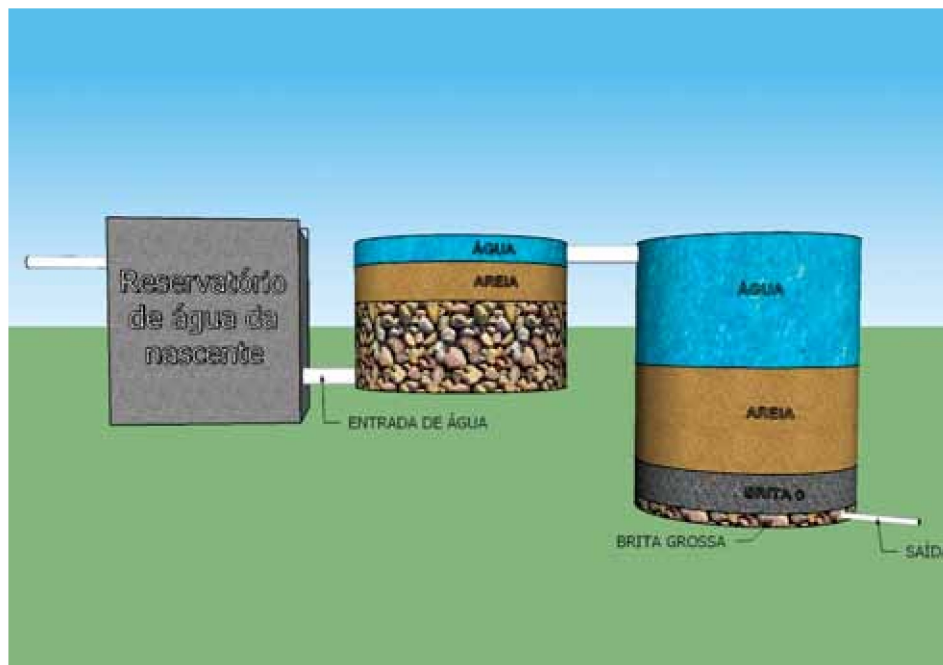
Esquema geral de filtragem de água de uma nascente
