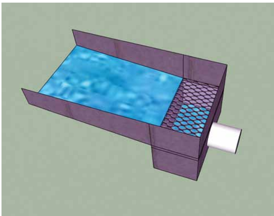
Calha com tela para pré-limpeza de impurezas
