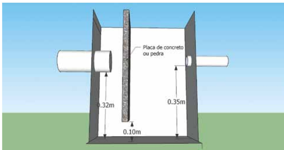
Corte lateral de uma caixa de gordura
