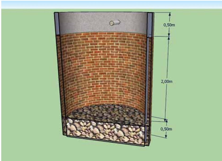
Vista lateral do sumidouro
