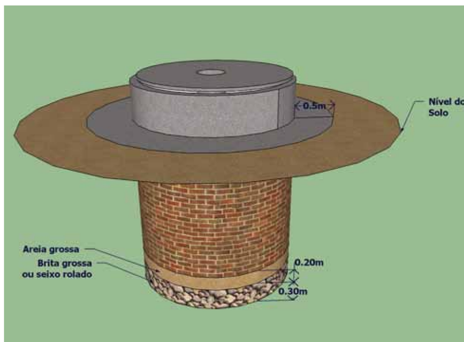
Esquema geral de construção de cisterna
