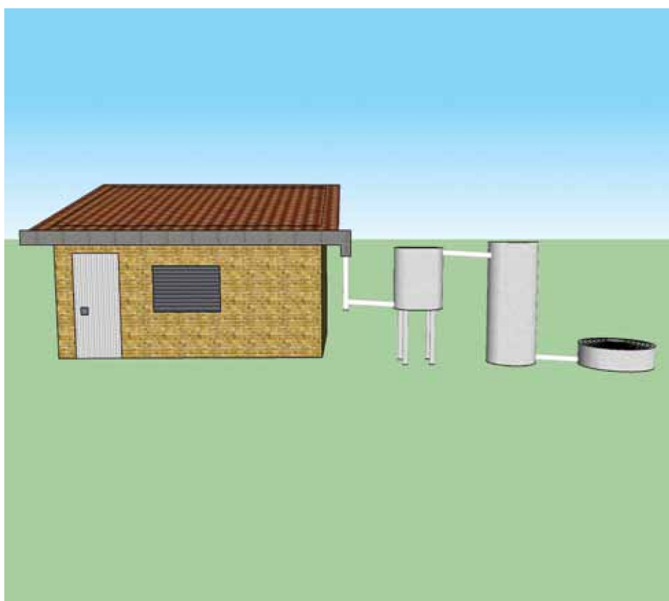
Esquema completo de coleta de água de chuva com filtro reservatório
