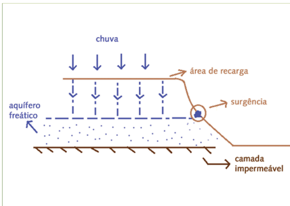
Esquema geral de nascentes
