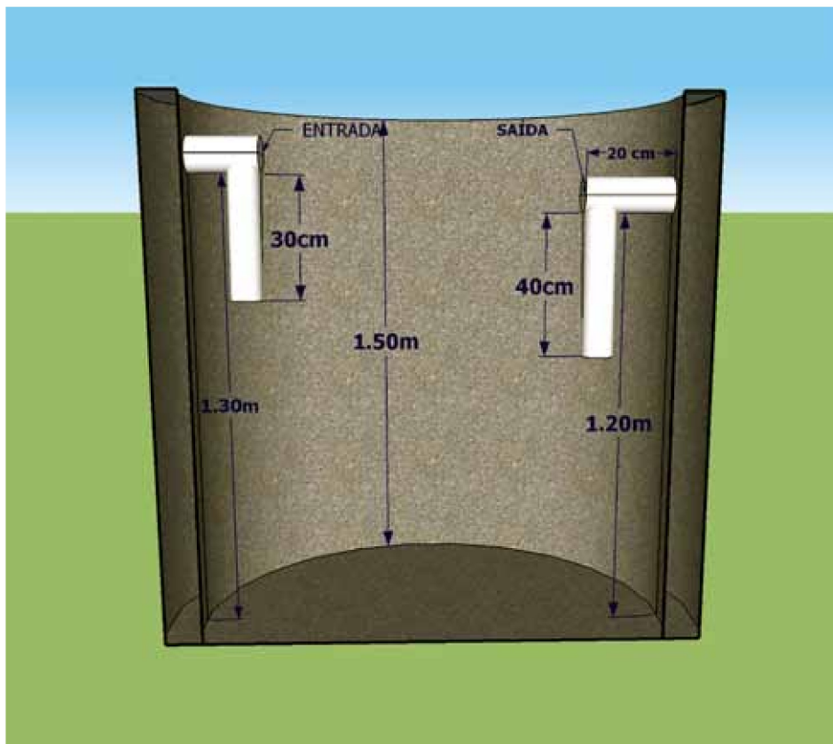
Vista lateral de fossa séptica circular sem divisões
