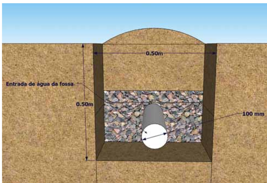
Detalhe de vala de infiltração
