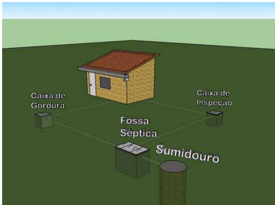
Esquema geral de um sistema de tratamento de efluentes
