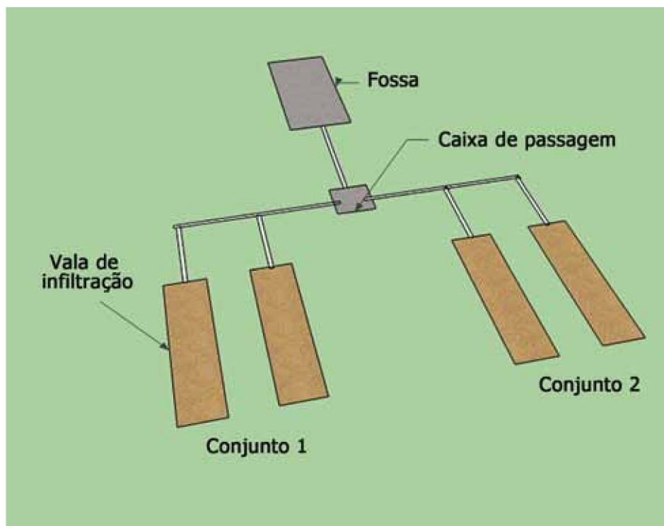
Esquema geral de valas de infiltração
