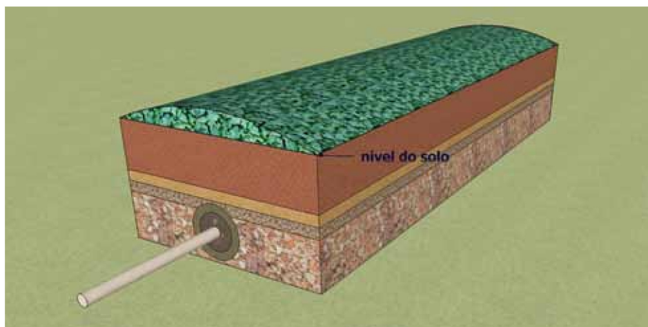
Vista geral de um tanque de evapotranspiração
