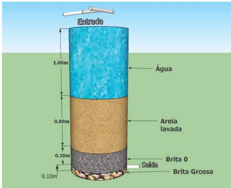
Esquema do interior do filtro
